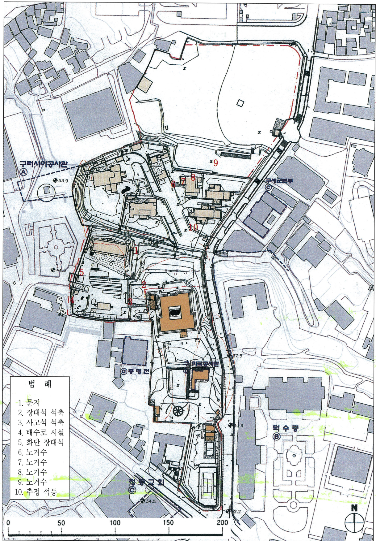
[도면 7] 조사지역내 유구·자연문화재 현황도
